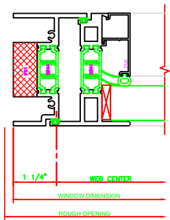
440 JAMB 325 CASEMENT OUT 4-BAR ARMS
